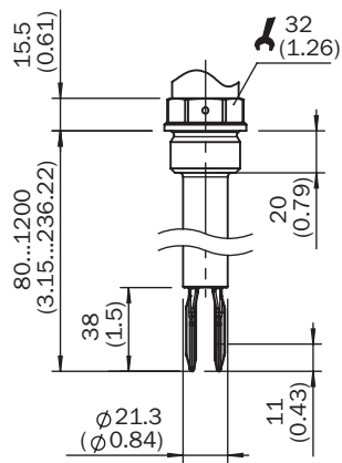
Габаритный чертеж корпуса
